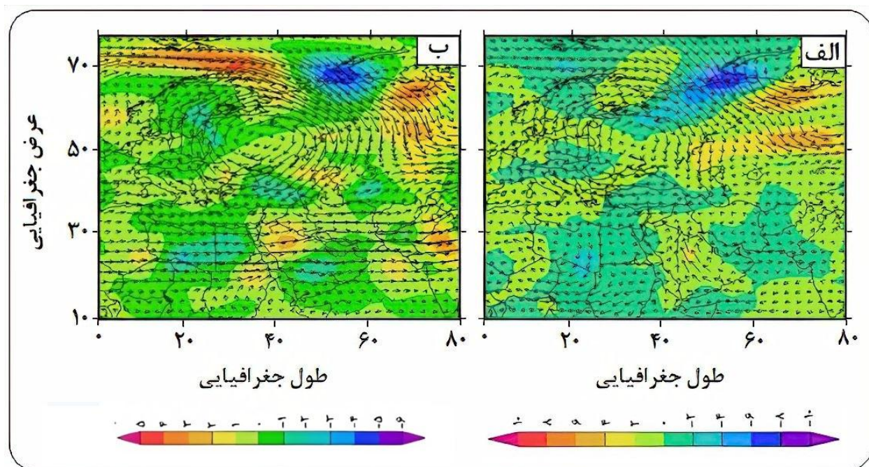
شکل ۵: فرافت دما و جهت جریان های هوا در ترازهای ۸۵۰ (الف) و ۵۰۰ (ب) هکتوپاسکال برای الگوی دوم
